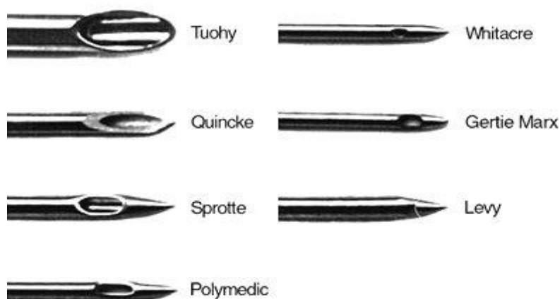
Figura No. 2 Diseños de agujas para punción neuroaxial
