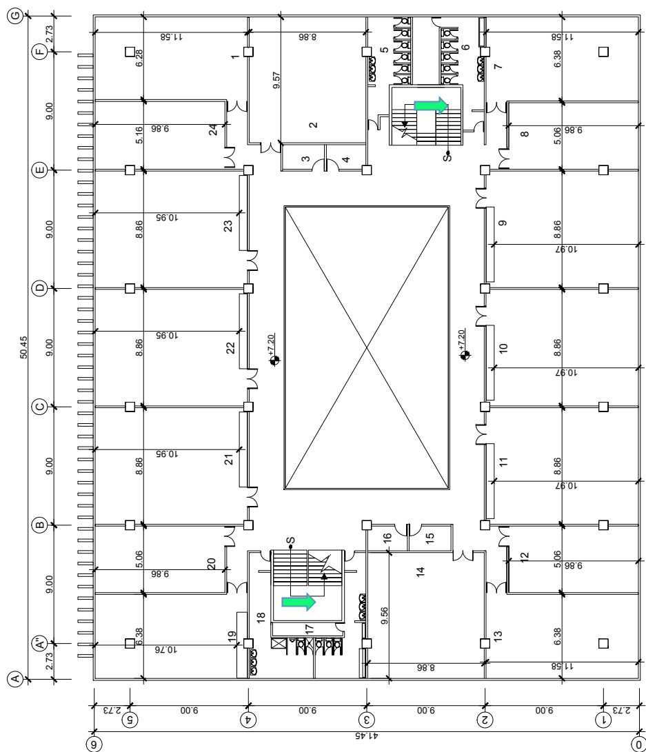
PLANTA AMUEBLADA TERCER NIVEL EDIFICIO DE MEDICINA "B"
